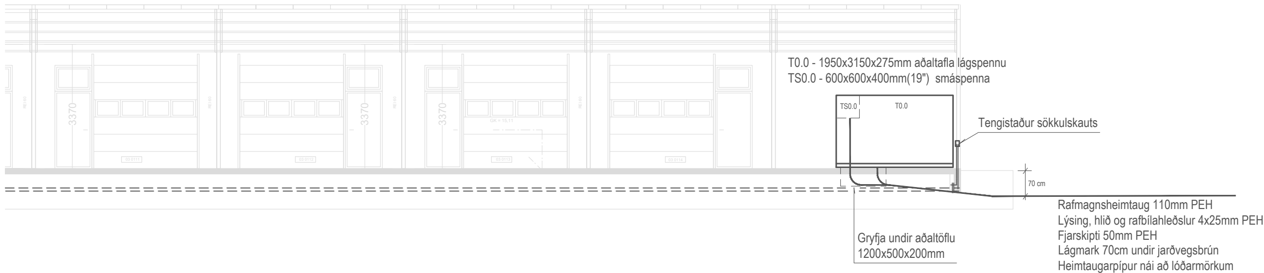
SNIÐ um inntak - M 1:100
